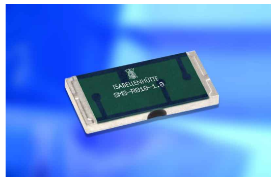
Bauform/Size 2512
