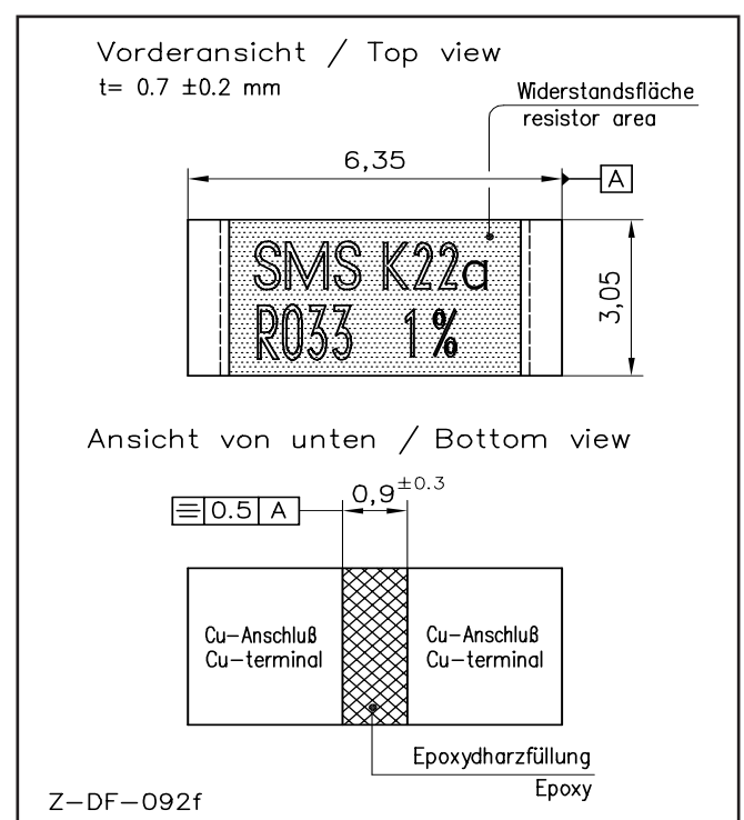
Bauform/Size 2512
