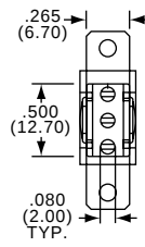
SPDT
