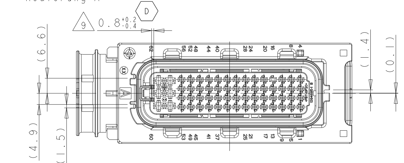
PRE LOCKED POSITION OF SECONDARY LOCKING Vorraststellung der 2. Kontaktsicherung CODING A Kodierung A
