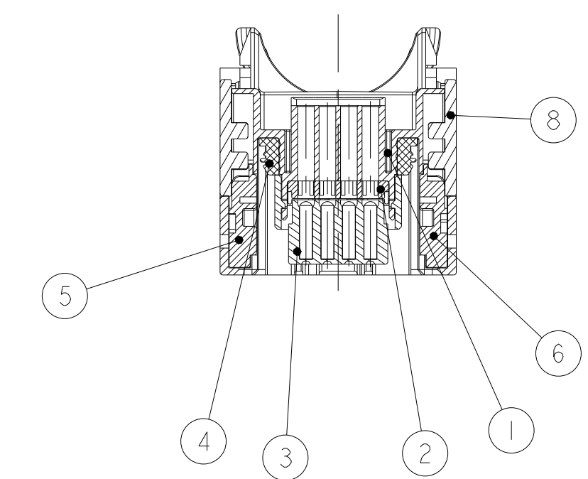
SECTION B-B Schnitt
