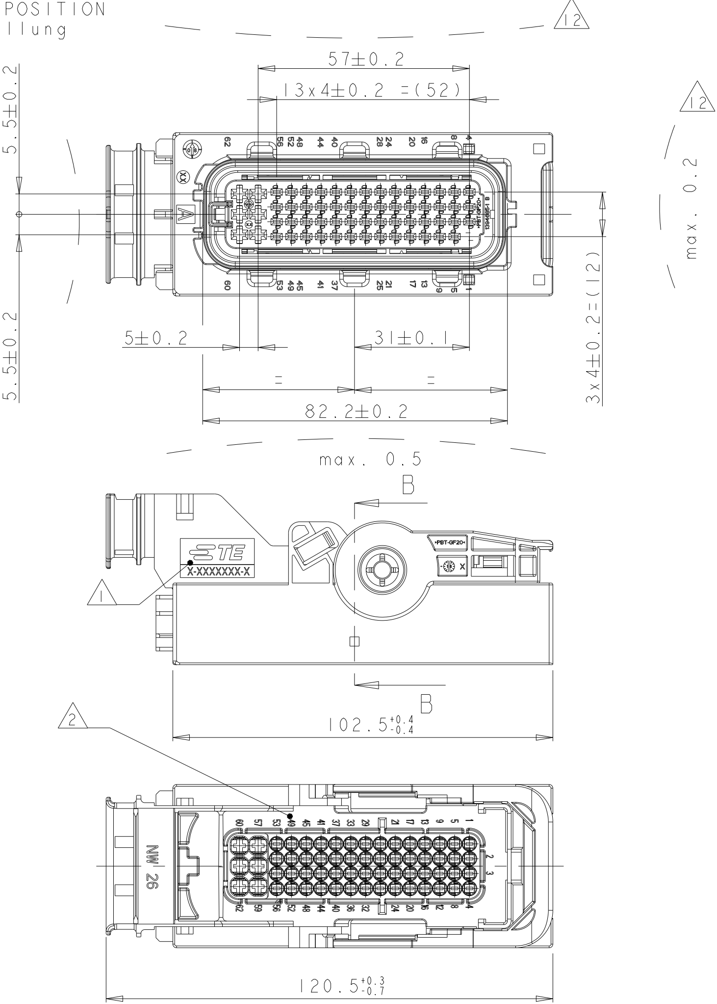
LEVER IN LOCKED POSITION Hebel in Verriegelungsstellung
