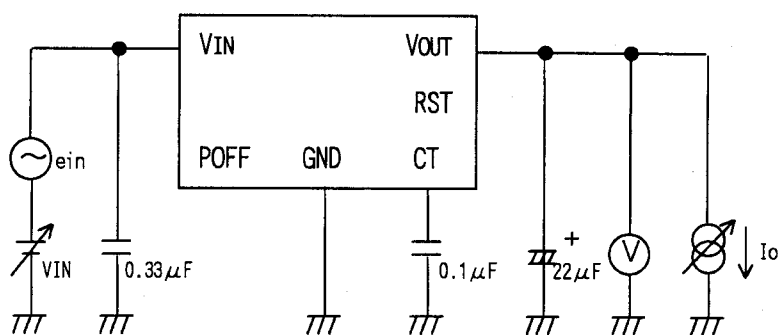
Measuring circuit for Ripple Rejection Ratio リップル リジエクション測定回路
