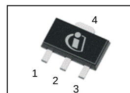
PG-SOT-89
