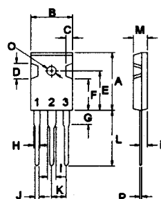
TO-247(3P)
