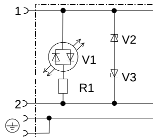
STROMLAUFPLAN Schematic diagram
