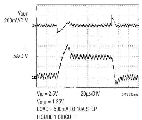
Load-Step Transient
