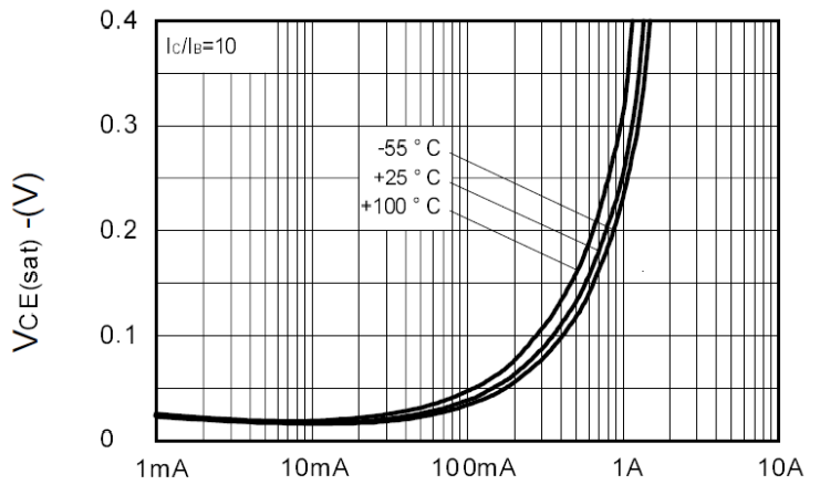
V_{CE(sat)} v I_C
