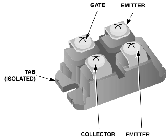
JEDEC STYLE SOT-227B
