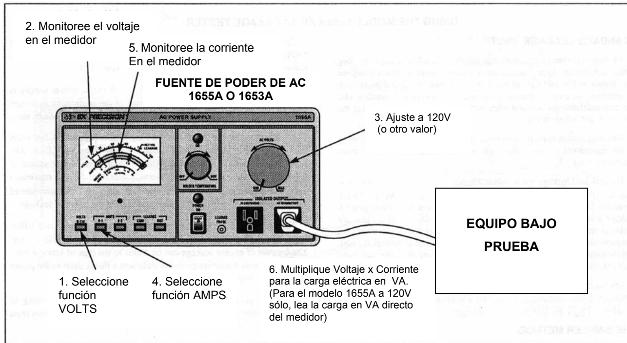
Fig. 11. Medición de carga eléctrica
