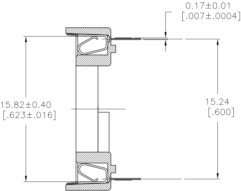
SECTION D-D
