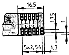
Printplatte lang für Dezimalausführung (Lötanschluß) Bestellbez. AL
