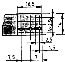
Printplatte lang Bestellbez. AL
