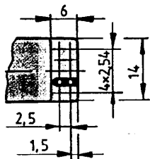
Printplatte kurz Bestellbez. AK
