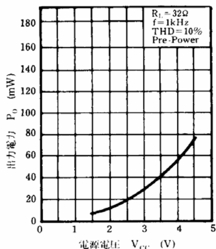
P_O - V_{CC}
