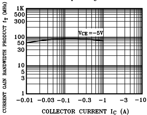
f_T - I_C
