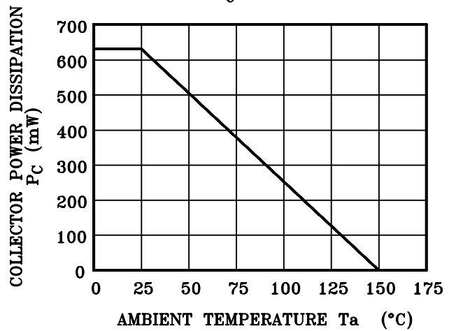
P_C - T_a
