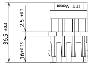
Receptacle, 3 poles
