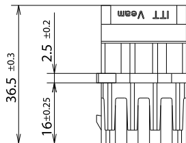
Receptacle, 6 poles
