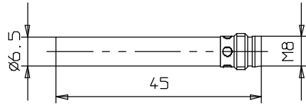
E2EL- C1R5□ - M3
