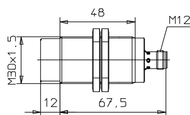
E2EL-X15M□-M1L
