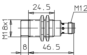
E2EL-X8M□-M1
