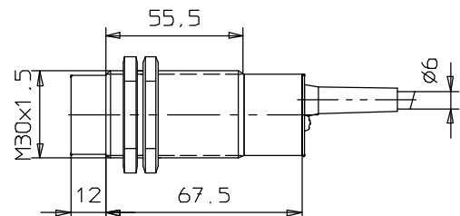
E2EL-X10□-L
