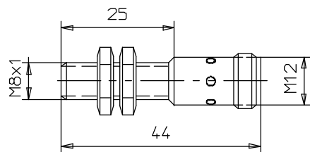
E2EL- X1R5□ - M1
