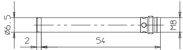
E2EL- C2M□ - M3L
