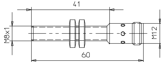
E2EL- X1R5□ - M1L
