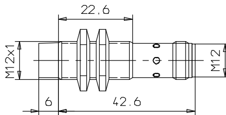
E2EL-X4M□-M1
