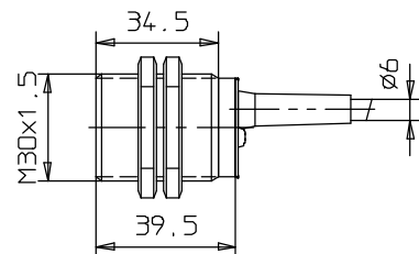
E2EL-X10□
