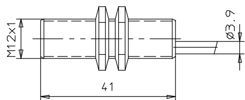
E2EL-X2□ 2M, E2EL-X4□-D 2M, E2EL-X4□-DS
