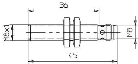
E2EL- X1R5□ - M3
