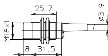
E2EL-X8M□
