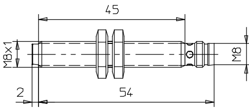
E2EL- X2M□ - M3L
