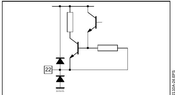
Figure 22 : Pin 22 (DLO)
