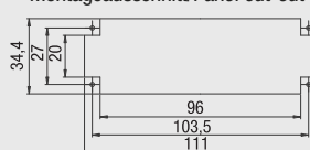
Montageausschnitt/Panel cut-out
