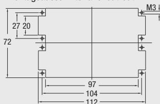
Montageausschnitt/Panel cut-out
