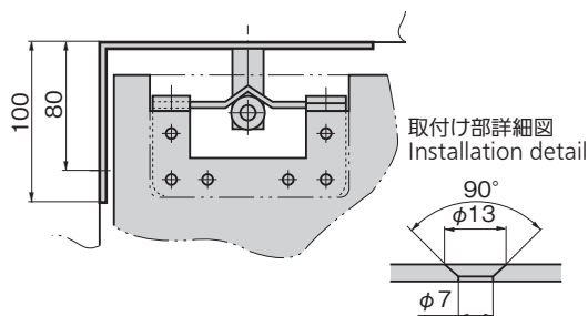
下部ヒンジ詳細図 Lower hinges detail
