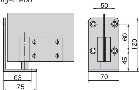
下部ヒンジ詳細図 Lower hinges detail
