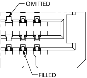
DETAIL 'G' SCALE 5:1
