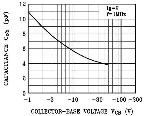
C_{ob} - V_{CB}
