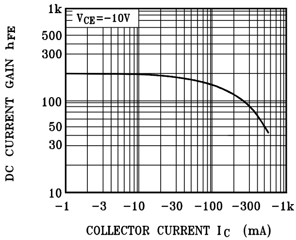
h_{FE} - I_C
