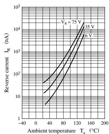
I_R - T_a
