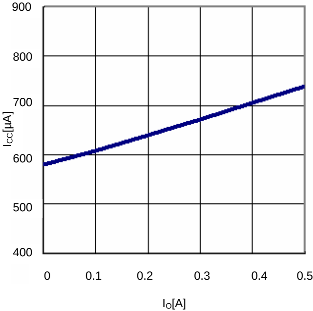
Fig.20 I_o - I_{cc}
