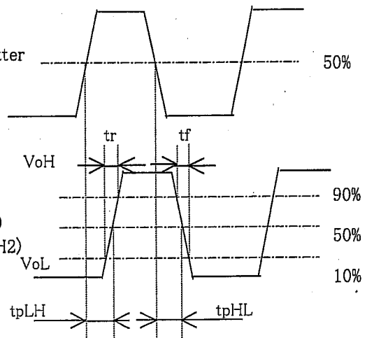
入力信号(CH1) Input signal(CH1)
