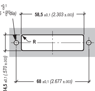
Perçage pour boîtier mâle à picots fixation sur panneau avec détrompeur réf. 001900 081 00 Cutout for pin contact receptacle fixation on panel with polarizer P/N 001900 081 00
