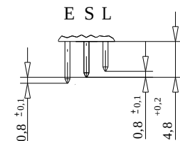
Stecklänge / mating length
