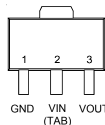
SOT-89
