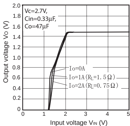
Fig.7 Output Voltage vs. Input Voltage (PQ015EZ02ZxH)
