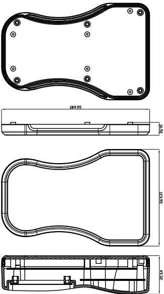
TOP-(NQ-LCD)
