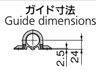
FA-1825N-2A A型フック A hook section
