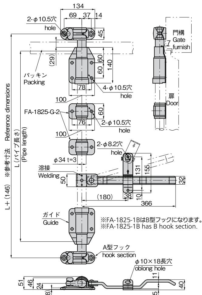
〔FA-1825N-1A〕ハンドル受け金具タイプ Handle receptor type
