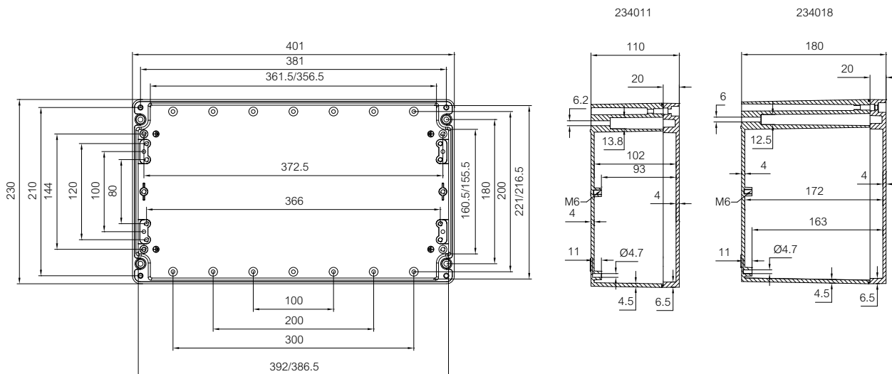
ALU 401x230x110-180
