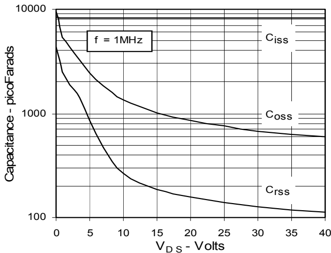
Fig. 11. Capacitance
