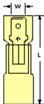
MNHU10-250DMI 12-10 MNHU10-250DFI
