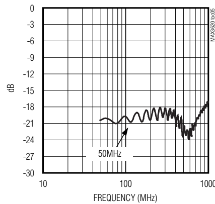
MAX3620A S11
