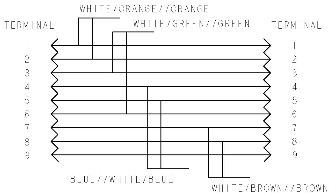
WIRING DIAGRAM 568B
