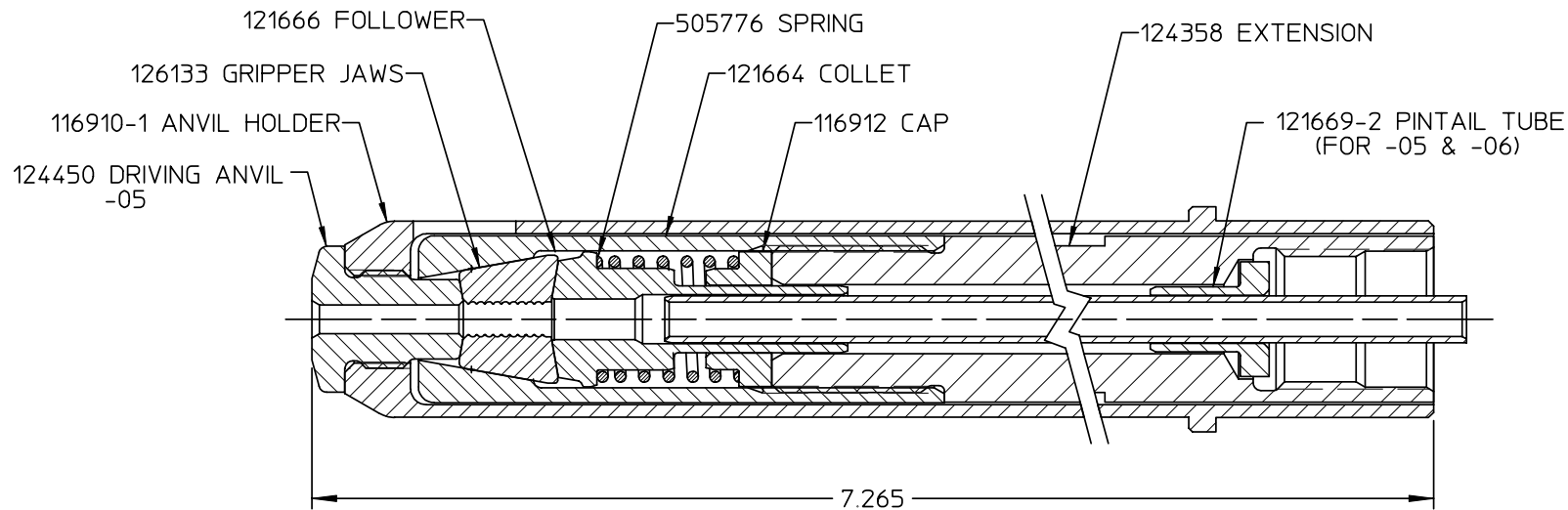
SECTION A-A
