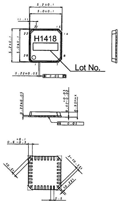
VQFN28 (Unit : mm)
