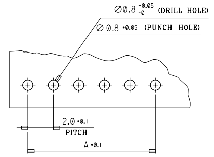
PC-BOARD LAY-OUT(t=1.6) (SCALE 5:1)
