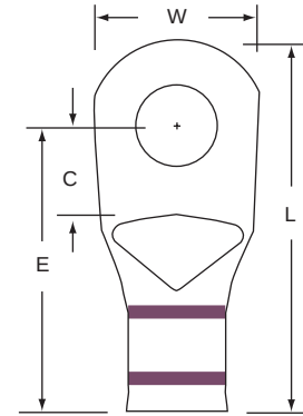
MC2-38RX Stud Size Wire Range 3/8 2
