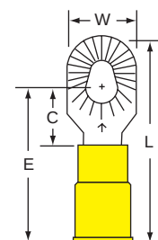
13-610-NB Stud Size Wire Range
