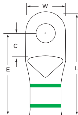
MC1-516RX Stud Size Wire Range 5/16 1
