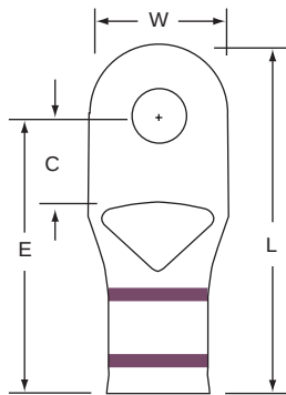
MC2-14RX Stud Size Wire Range 1/4 2
