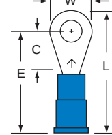
L-12-8-P Stud Size 8 Wire Range 16-14
