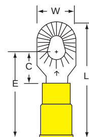
13-610-P Stud Size Wire Range
