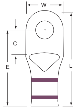
MC2-516RX Stud Size Wire Range 5/16 2
