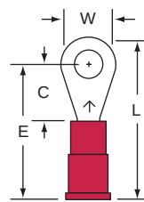
L-11-8-P Stud Size Wire Range 8 22-18
