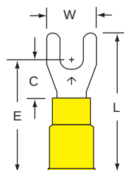
33-8-P Stud Size 8 Wire Range 12-10
