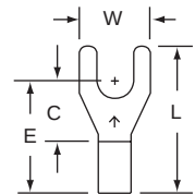
32-10-W Stud Size 10 Wire Range 16-14
