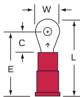
11-2S-P Stud Size Wire Range 2 22-18
