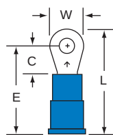
12-4S-P Stud Size 4 Wire Range 16-14
