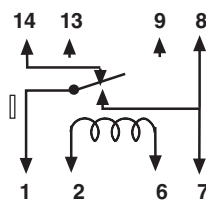
SPDT
