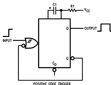
POSITIVE EDGE TRIGGER
