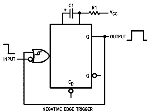
NEGATIVE EDGE TRIGGER
