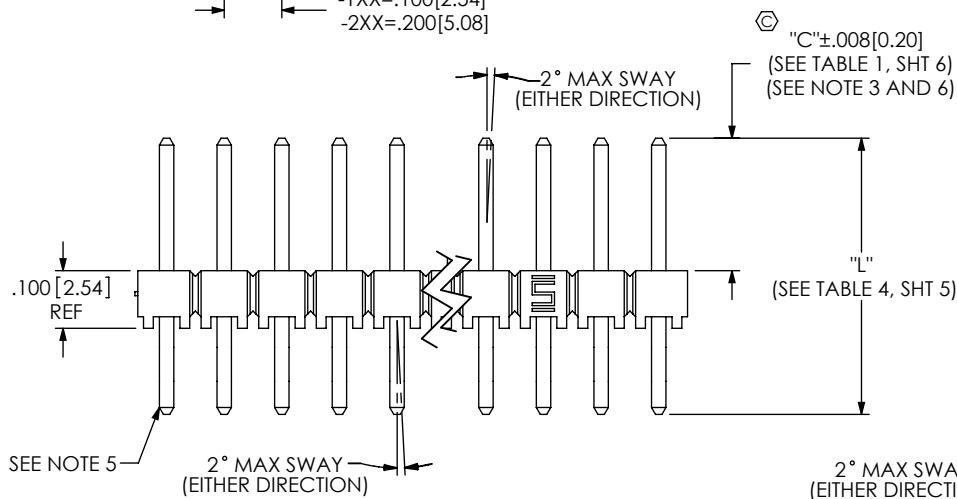
FIG 1 (TSW-1XX-XX-XX-S SHOWN)
