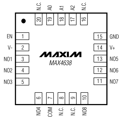
QFN
