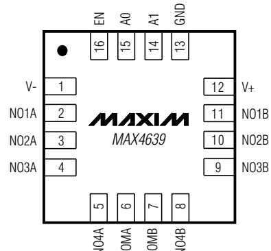
QFN
