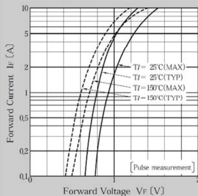
順方向特性
