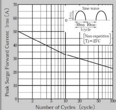
せん頭サージ順電流耐量
