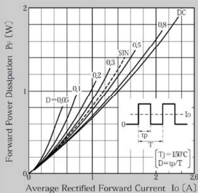
順電力損失曲線
