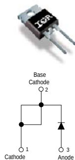
TO-220AC
