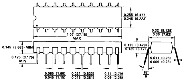
20-Pin Plastic DIP (N-20)
