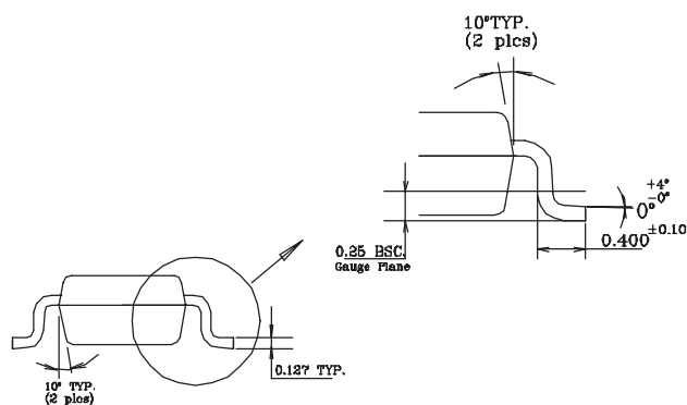
TSOT-23-5 (D5)
