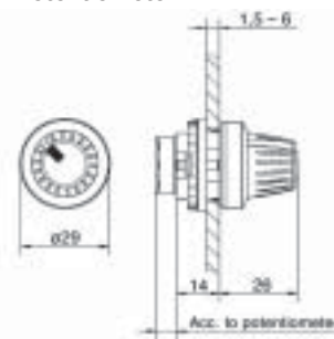
Potentiometer
