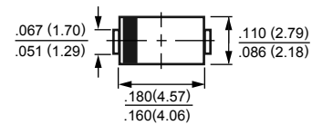
DO214AC(SMA)
